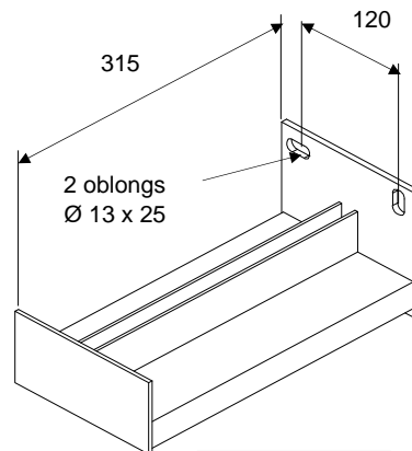
Console S 39-DS (code 095603) Poids : 4,10 kg
