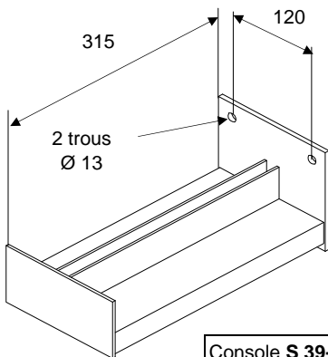
Console S 39-D (code 095602) Poids : 4,10 kg
