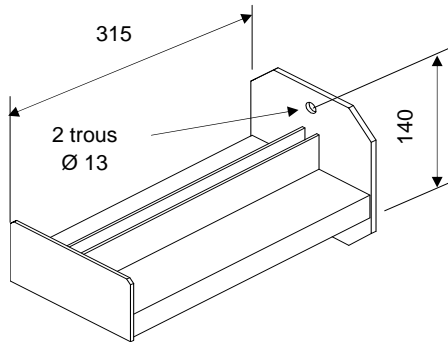
Console S 38 (code 095600) Poids : 4,10 kg
